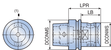
HSK DIN 69893-E MB
