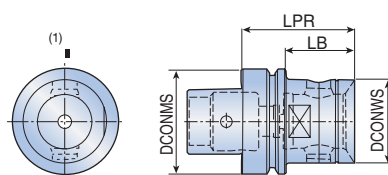
HSK DIN 69893-F MB
