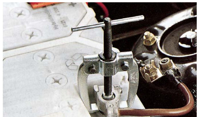
ściągacz do zdejmowania biegunów akumulatorów
