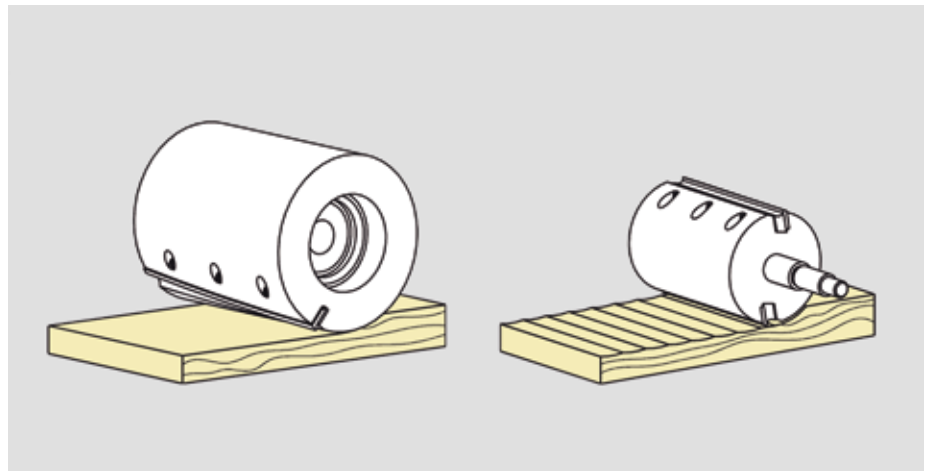
Bezkonkurencyjna koncepcja noża spiralnego Spir-O-Cut: cięcie ruchem koszącym zapewnia gładkie powierzchnie ze zminimalizowanymi śladami obróbki – przy jednocześnie wyciszzonej pracy.
